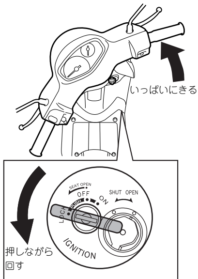
ハンドルロックのかけかた
