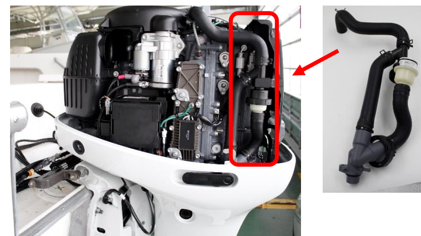
マイクロプラスチック回収装置
