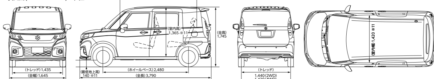
寸法図(HYBRID MZ) 単位:mm
